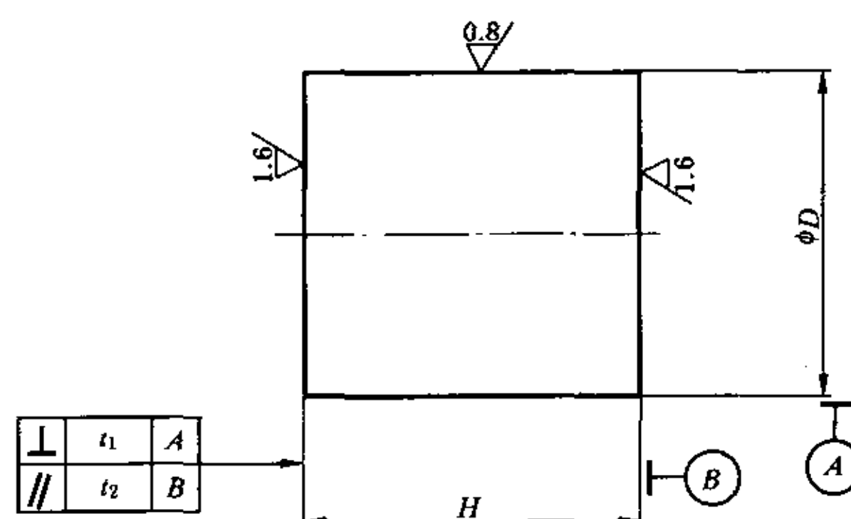
图 1 圆形镶块
